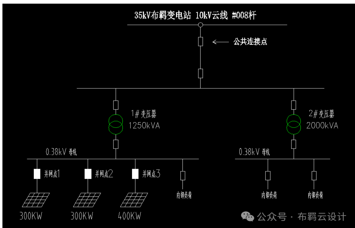
图三 三个并网点，一个接入点
