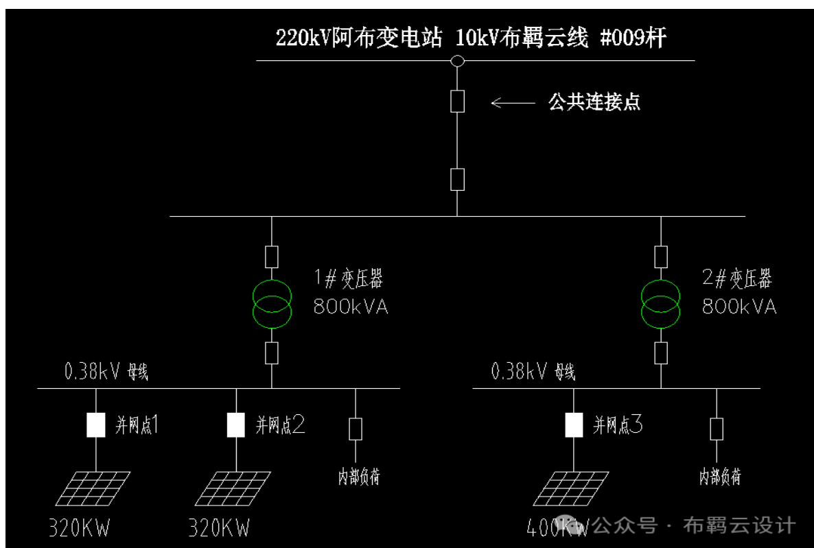
图一 三个并网点，三个接入点
