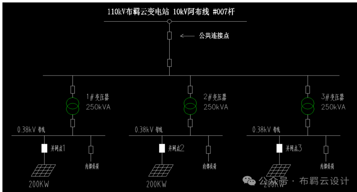
图一 三个并网点，三个接入点
